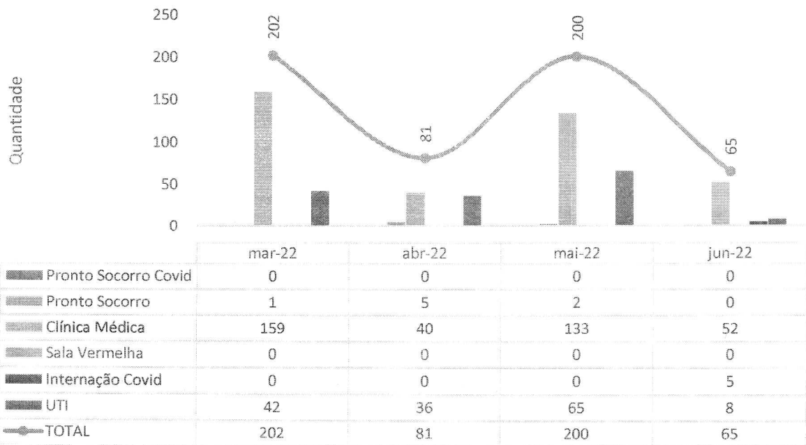
HETRIN - atendimentos de Fonoaudiologia por Clínica - Jun-22
